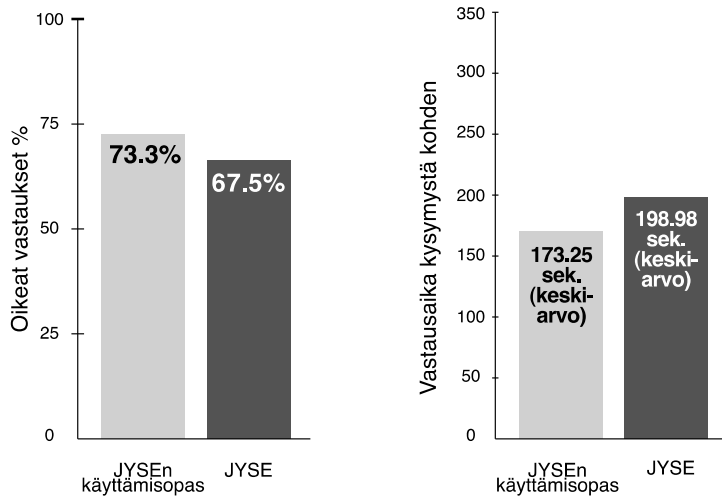
Kuva 1: Ymmärtämistehtävien tuloksia
