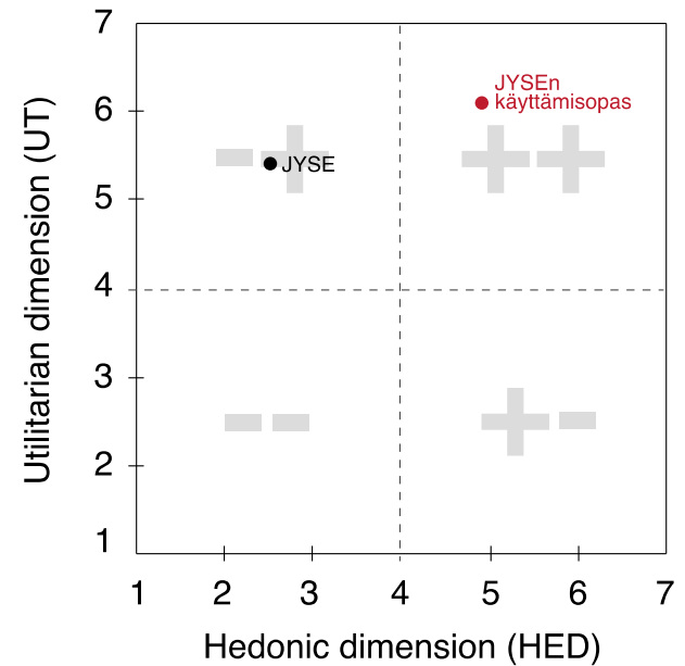
Kuva 2: Käytön arviointituloksia
